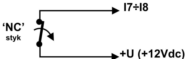
Wejście (I7,I8) w konfiguracji: NO wyzwalane przez +12V, zdjęta zworki JI7,JI8.
